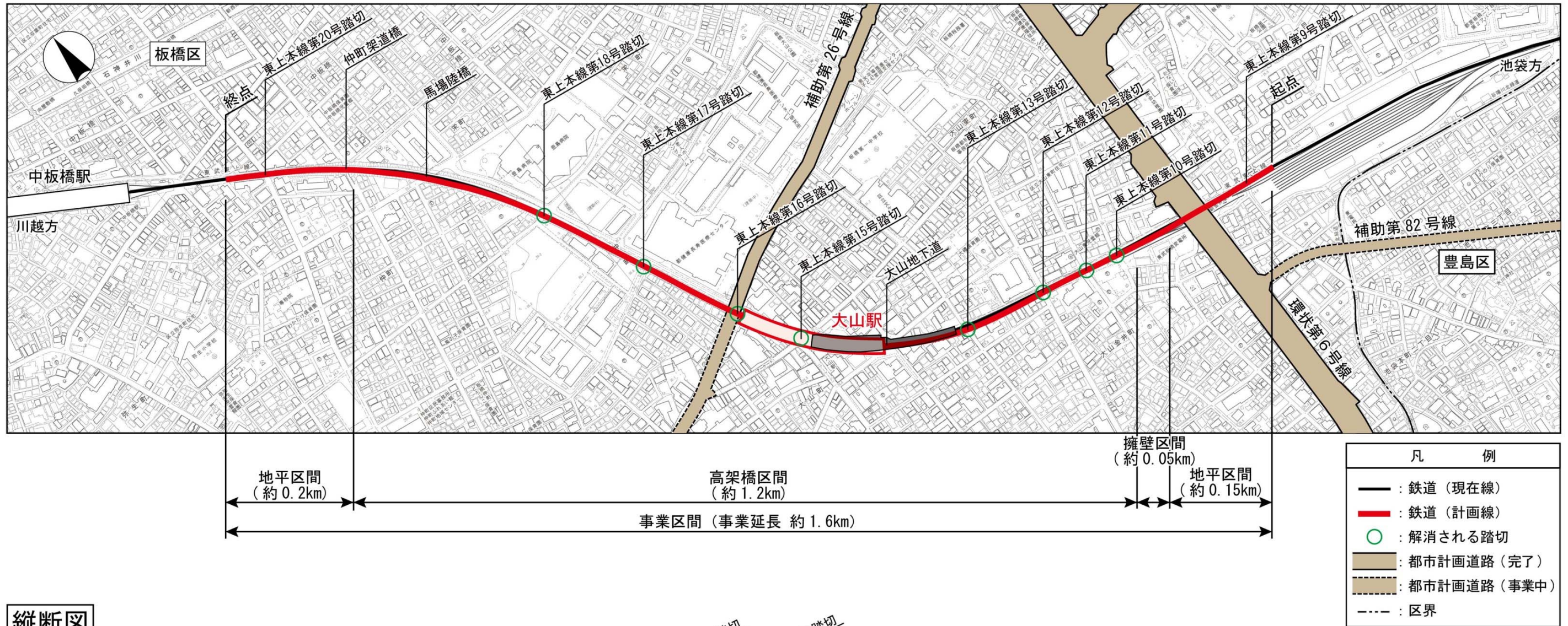
平面図
